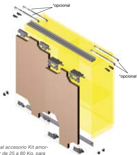
Montaje puerta interior
