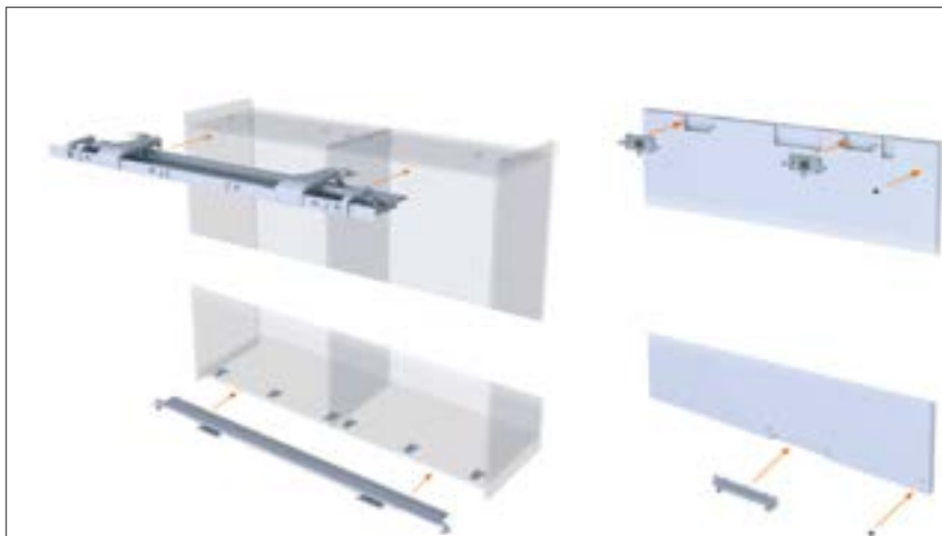
Patas frontales niveladoras incluidas en la guía inferior con su tapa
