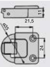
31.0441.3 Bisagra para patín.
