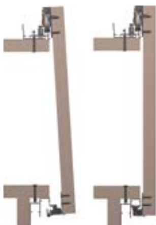
Montaje puerta interior
