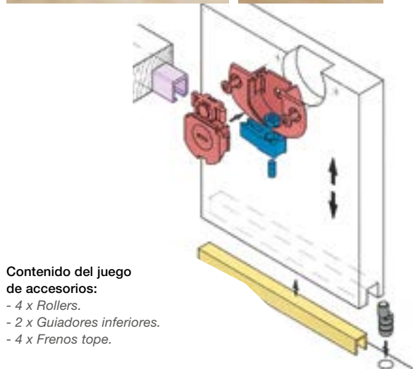
39.1223.2 Juego de accesorios corredera, 15 Kg. para 2 hojas mueble.
