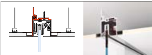
Instalación falso techo
