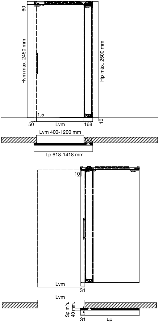
Sin guías ni guidores en el suelo
