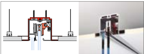
Instalación oculta falso techo
