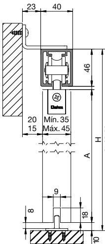
Guía STAR XL + Escuadra 55 mm.
