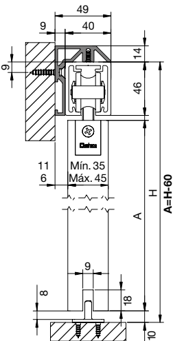
Guía STAR XL + Perfil separador
