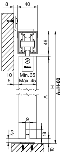
Guía STAR XL + Escuadra 40 mm.
