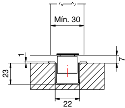
Montaje a suelo de guía inferior + guiador
