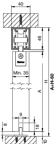
Guía STAR XL
