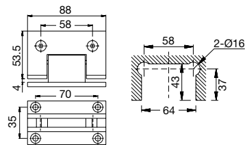
Bisagra apertura 180° fijación en pared Acero Inox AISI 304
