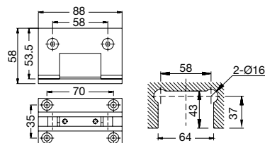
Fijación vidrio a pared con pletina Acero Inox AISI 304
