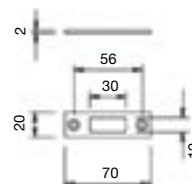
Cerradero fijación en pared Acero Inox AISI 304
