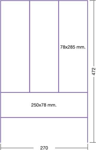
Medida del hueco del cubertero A
