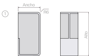
Sin pestaña y punto redondo
