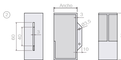
Con pestaña centradora y cantos rectos
